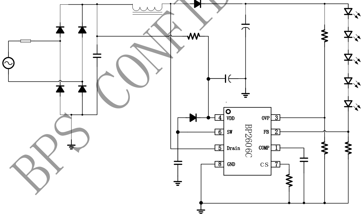
图 1 BP2606C 恒流典型应用图
