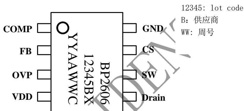
图 3 管脚封装图
