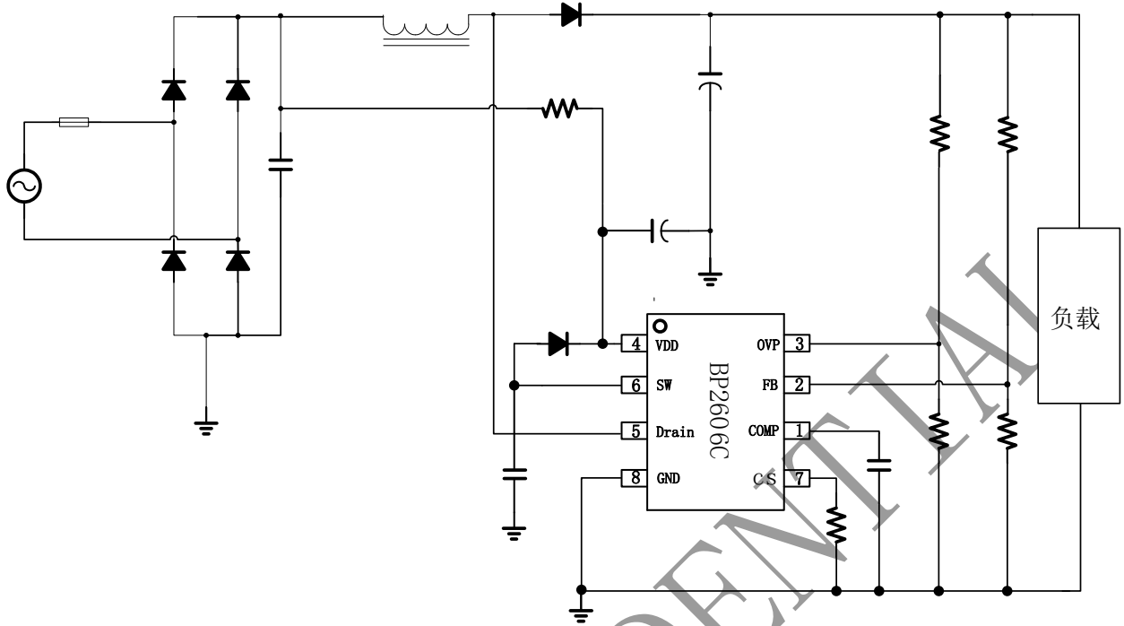
图 2 BP2606C 恒压典型应用图
